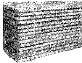
แผ่นพื้นคอนกรีตอัดแรง TRC 35 ซม. ขนาดลวด 4 มม.
